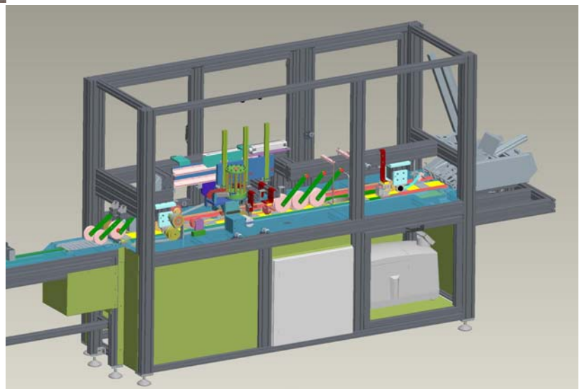
Detail: Papierstapel ausrichten, Fluttermarken prüfen, Dickenmessung
