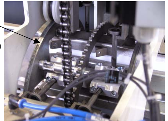
Detail aus Wendestation
