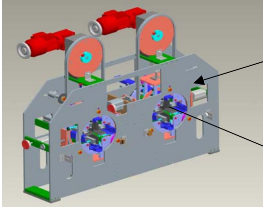
Wendestation in Kollationiermaschine
