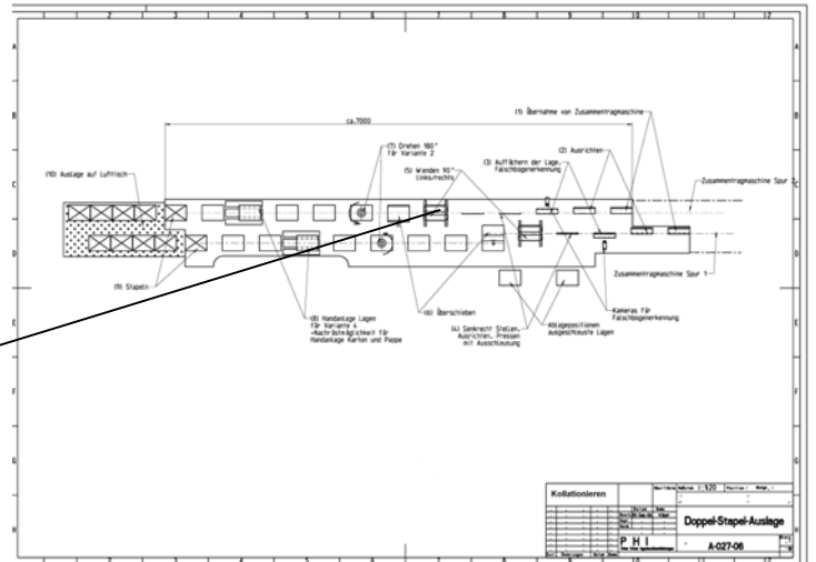
Wendestation in Kollationiermaschine
