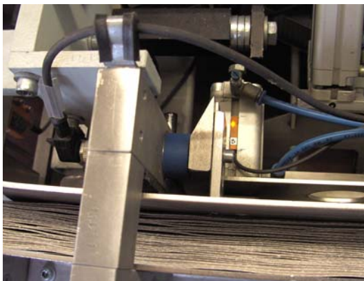
Detail: Papierstapel ausrichten, Fluttermarken prüfen, Dickenmessung
